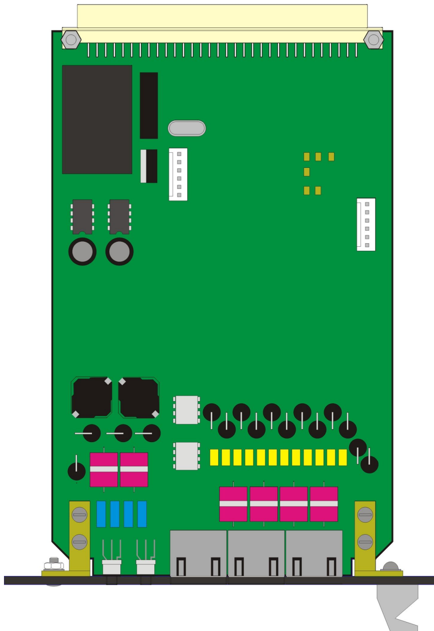
Внешний вид карты расширения V1A2 - МХ
