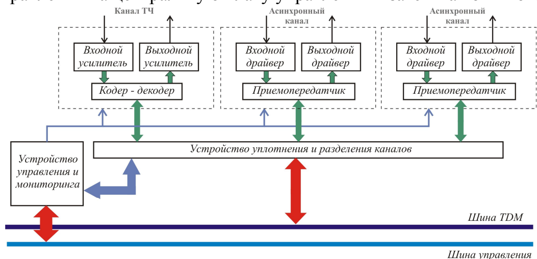
Рисунок 1 - Структурная схема карты расширения V2A1 - МХ
