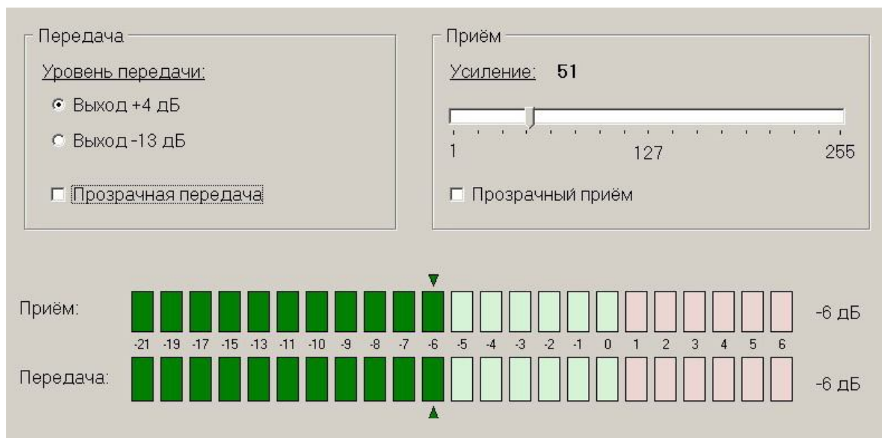
Рисунок 12 - Настройка канала ТЧ и индикация уровней сигналов
