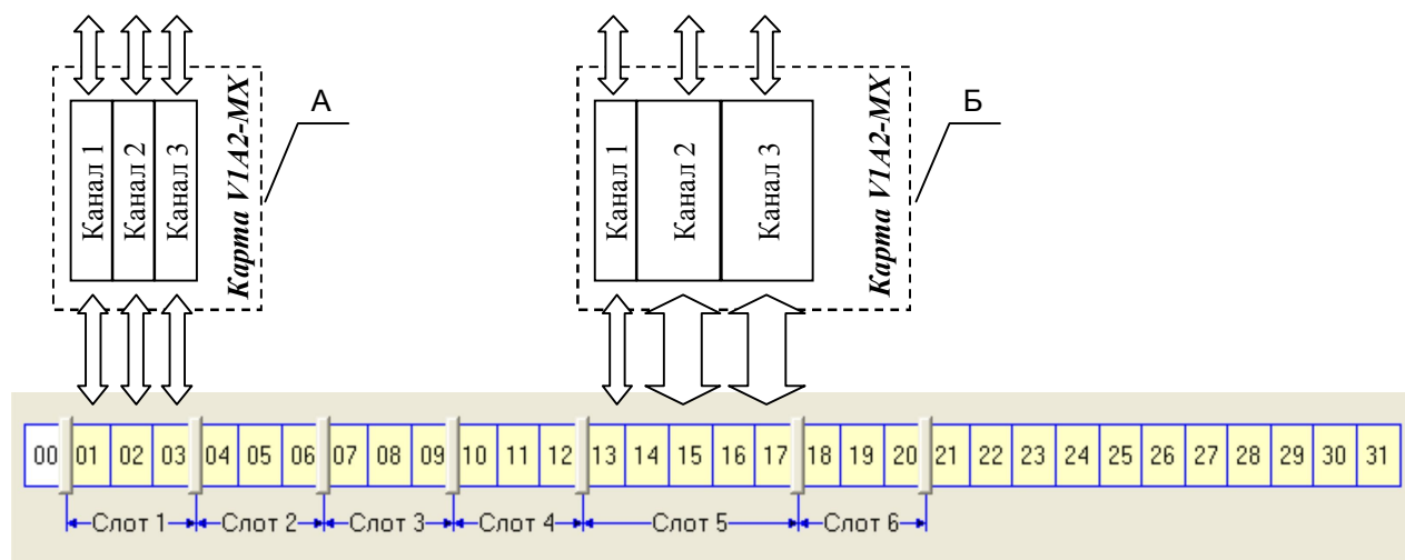
Рисунок 4 - Пример соответствия канальных интервалов для карт V1A2-MX, где А – асинхронные каналы работают в диапазоне скоростей 300...57600 бит/с, Б - асинхронные каналы работают со скоростью 115200 бит/с.
