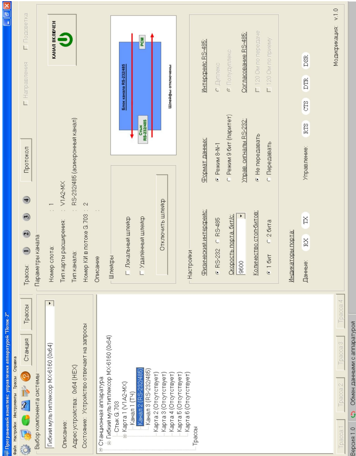
Окно ПО “Параметры асинхронного канала”
