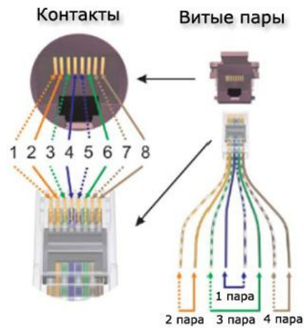
Рисунок 3 - Разводка проводов витой пары на разъем RJ-45
