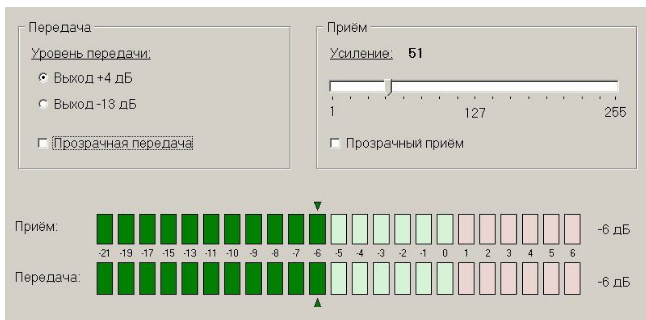
Рисунок 12 - Настройка канала ТЧ и индикация уровней сигналов
