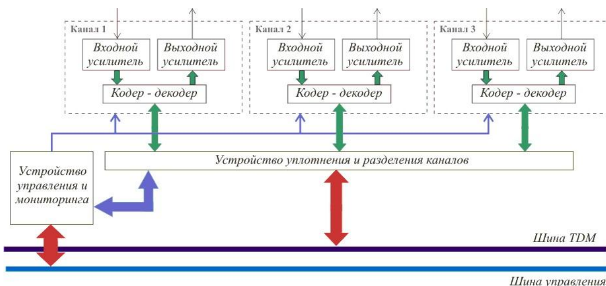
Рисунок 1 - Структурная схема карты расширения V3 - MX
