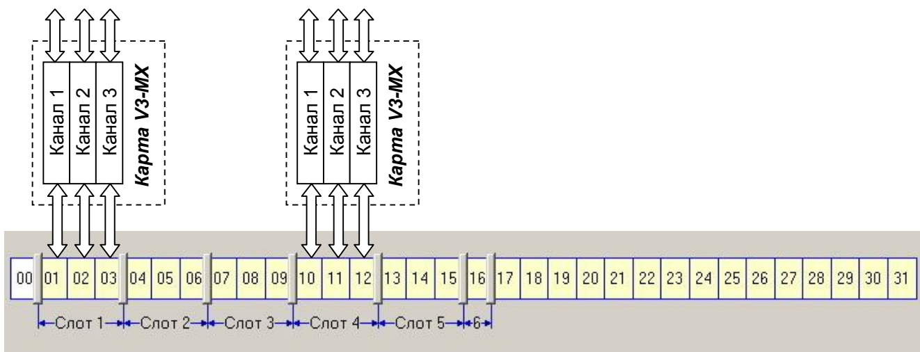
Рисунок 4 - Пример соответствия канальных интервалов для карт V3-MX
